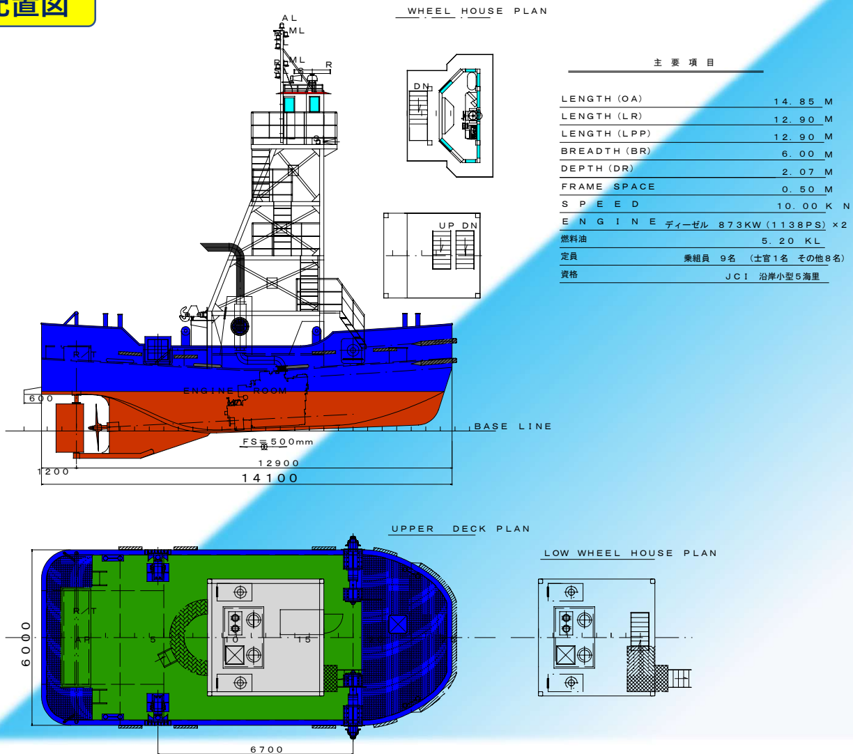
配置図
